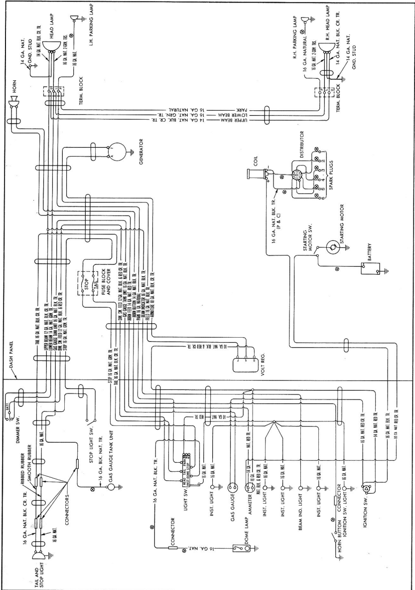
Fig. 2—(1950-51) Wiring Diagram
