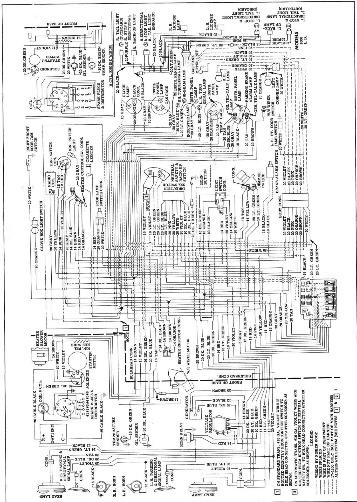
Fig. 16—Wiring Diagram—1959 Only
