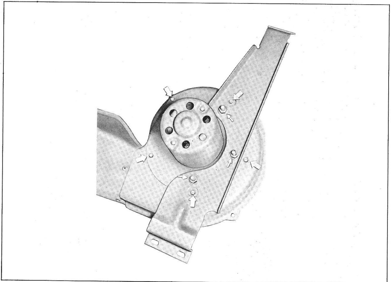
Fig. 36—Fan Motor Replacement—1960
