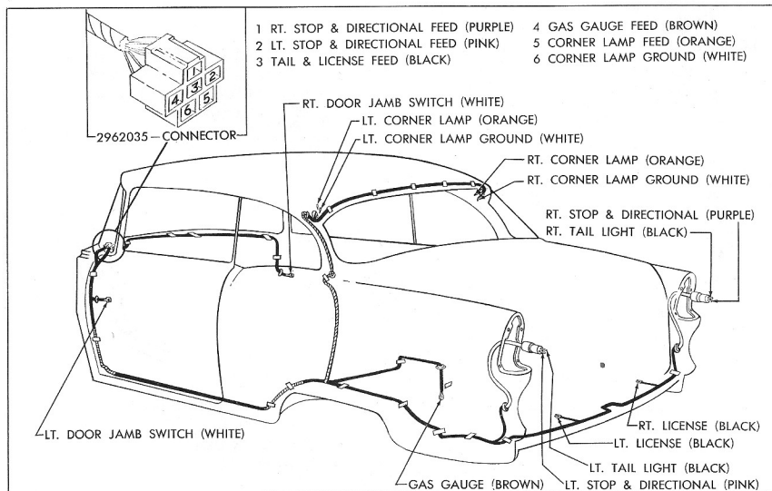
Fig. 123—Sport Coupe Wiring Diagram
