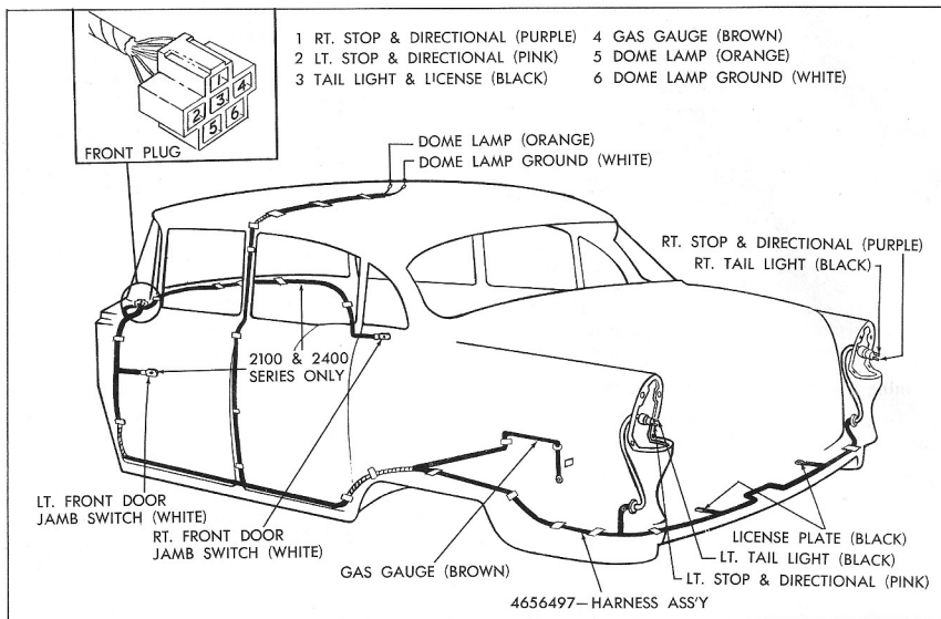
Fig. 122—Four Door Sedan Wiring Diagram
