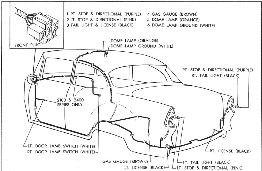
Fig. 124—Two Door Sedan Wiring Diagram
