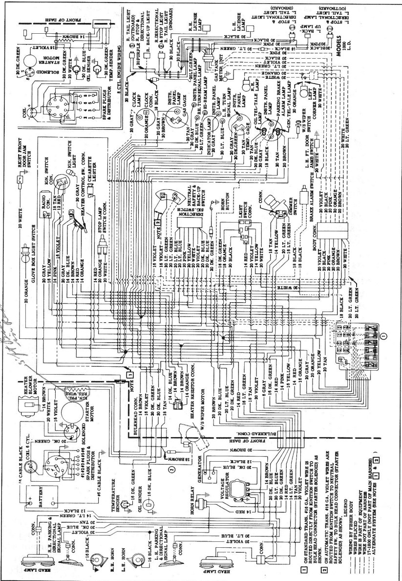
Fig. 18—1959 Wiring Diagram
